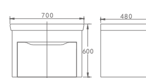
FH 9677 主柜 Main Cabinet 规格 Size:700 × 600 × 480
